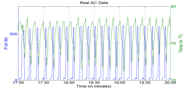
Fig. 5. Actual AC unit measurement data.
